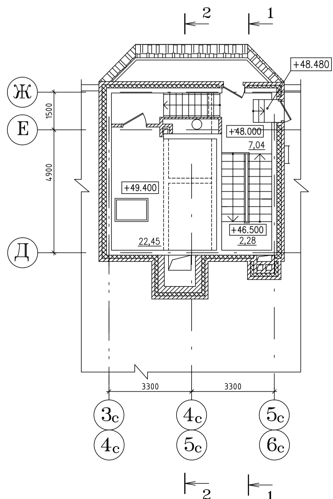
План машинного помещения лифтов
