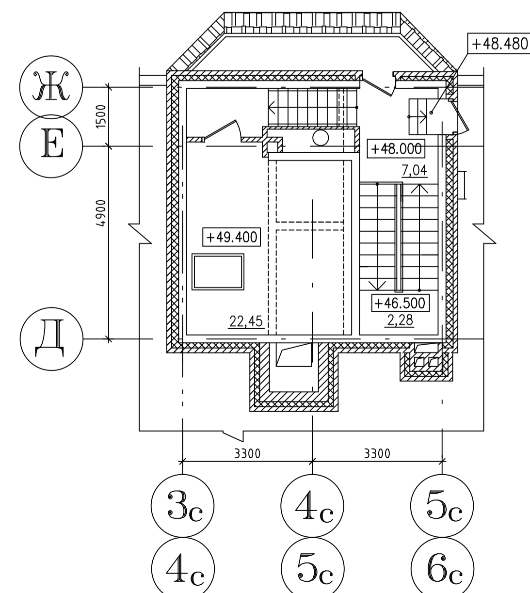
План машинного помещения лифтов
